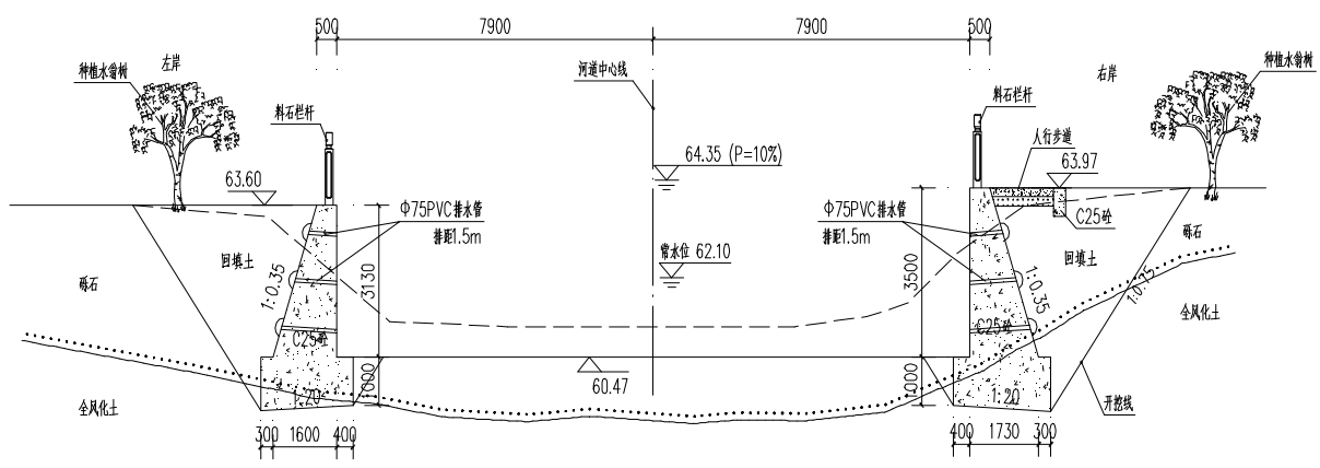
图 2.3-1 干流护岸代表断面图一
