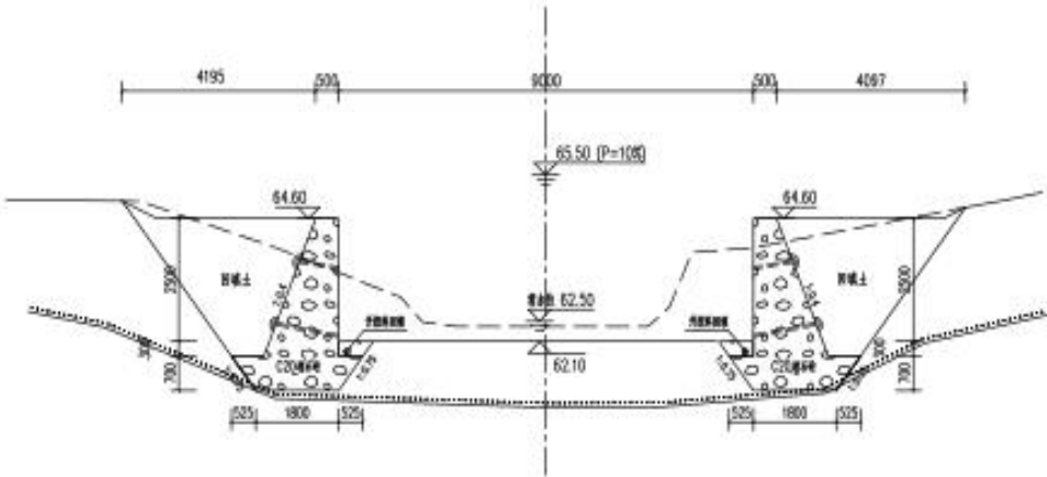
图3.2-1：直立式挡墙护岸典型剖面图
