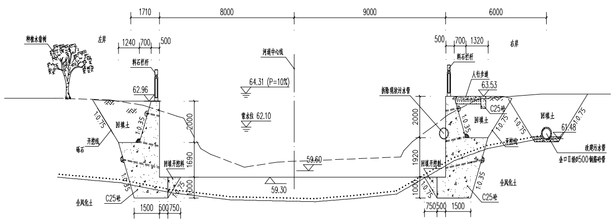
图 2.3-2 干流护岸代表断面图二
