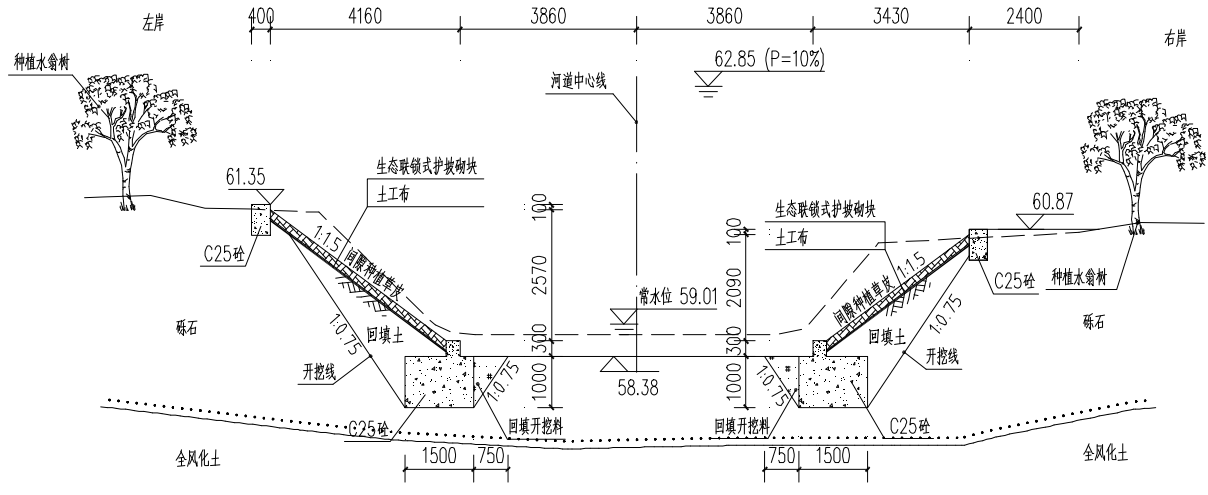
图 2.3-3 干流护岸代表断面图三
