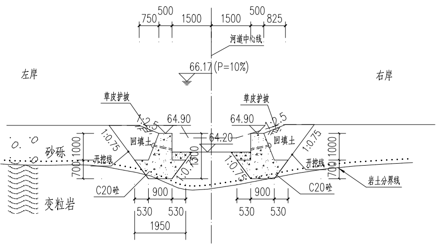
图 2.3-5 支流护岸代表断面图二
