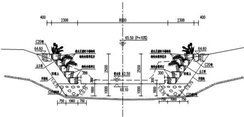
图3.2-2：阶梯式挡墙护岸典型剖面图
