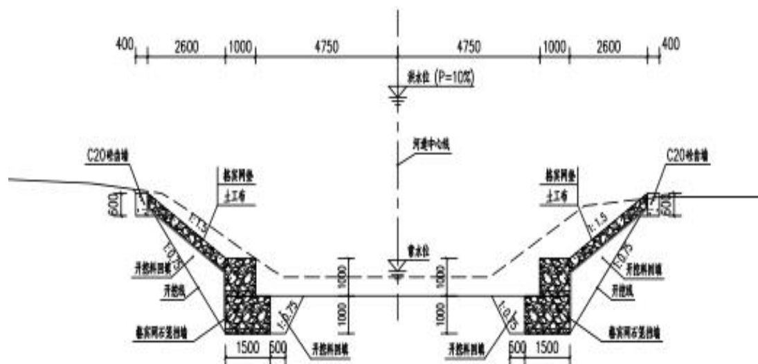
图3.2-3: 格宾网笼结构护岸典型剖面图
