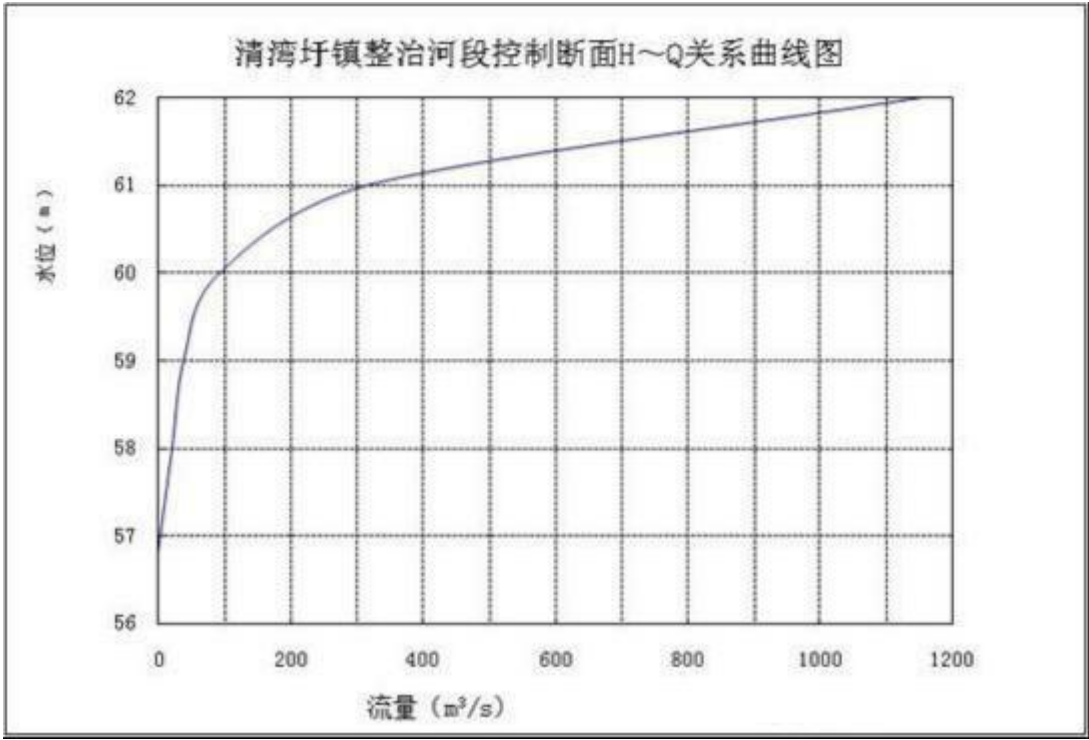
图 4.1-1：清湾圩镇整治河段下游控制断面 H~Q 关系曲线图
