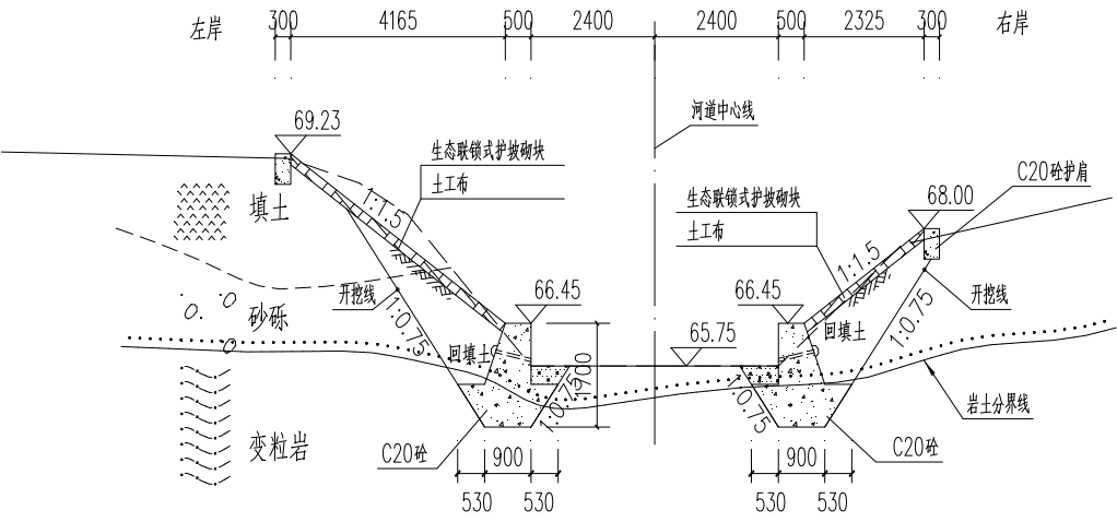
图 2.3-4 支流护岸代表断面图一
