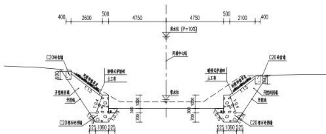
图3.2-4: 混凝土结构护岸典型剖面图
