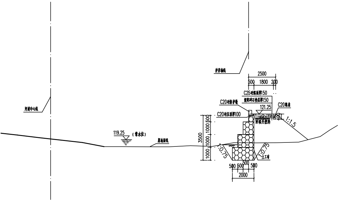
图 2.3-1 代表断面一
