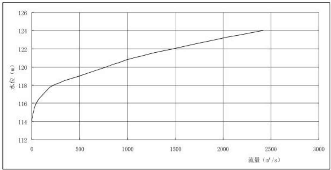
图 4.1-1 整治河段下游断面水位~流量关系曲线图
