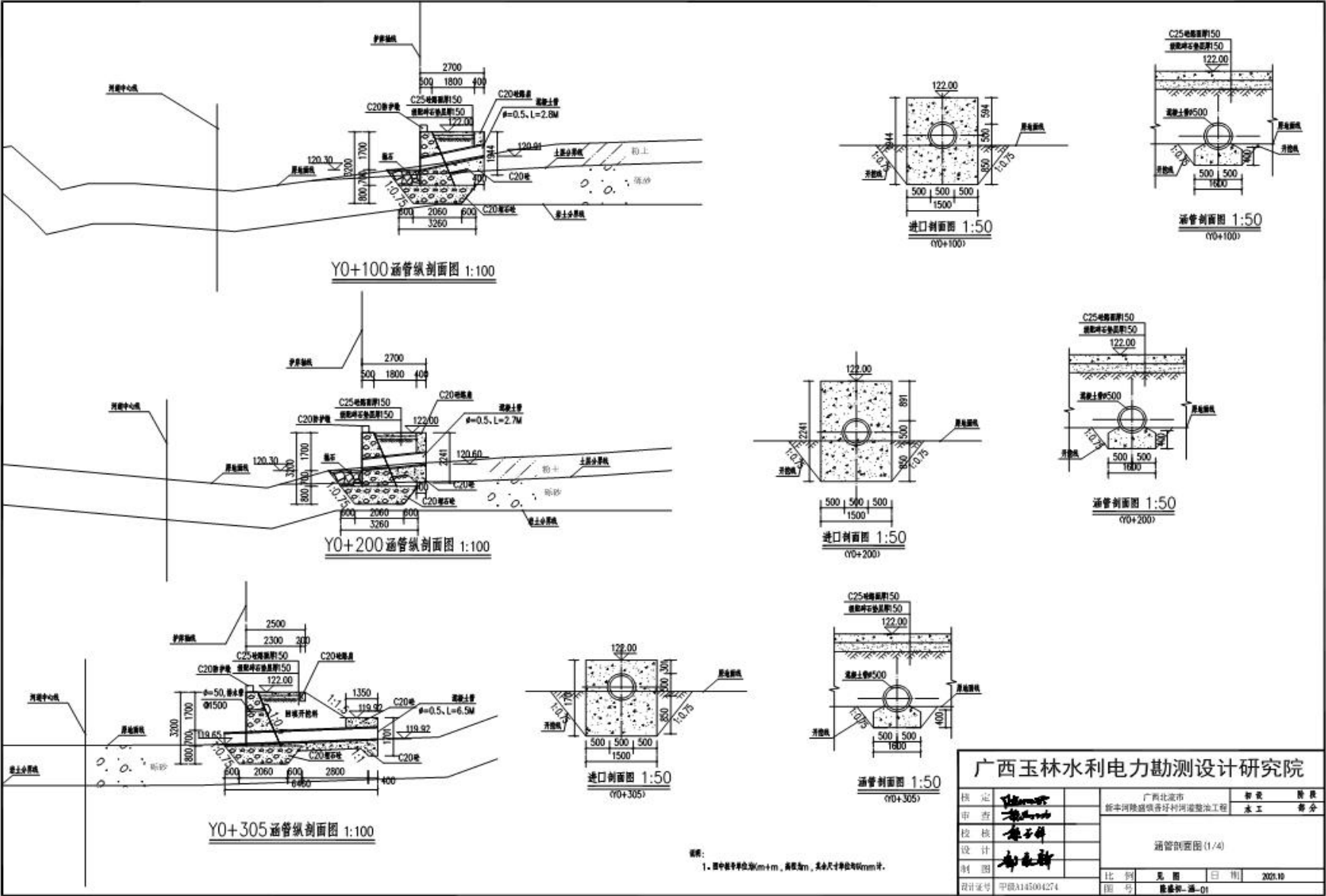
图 2.3-4 排水管设计图
