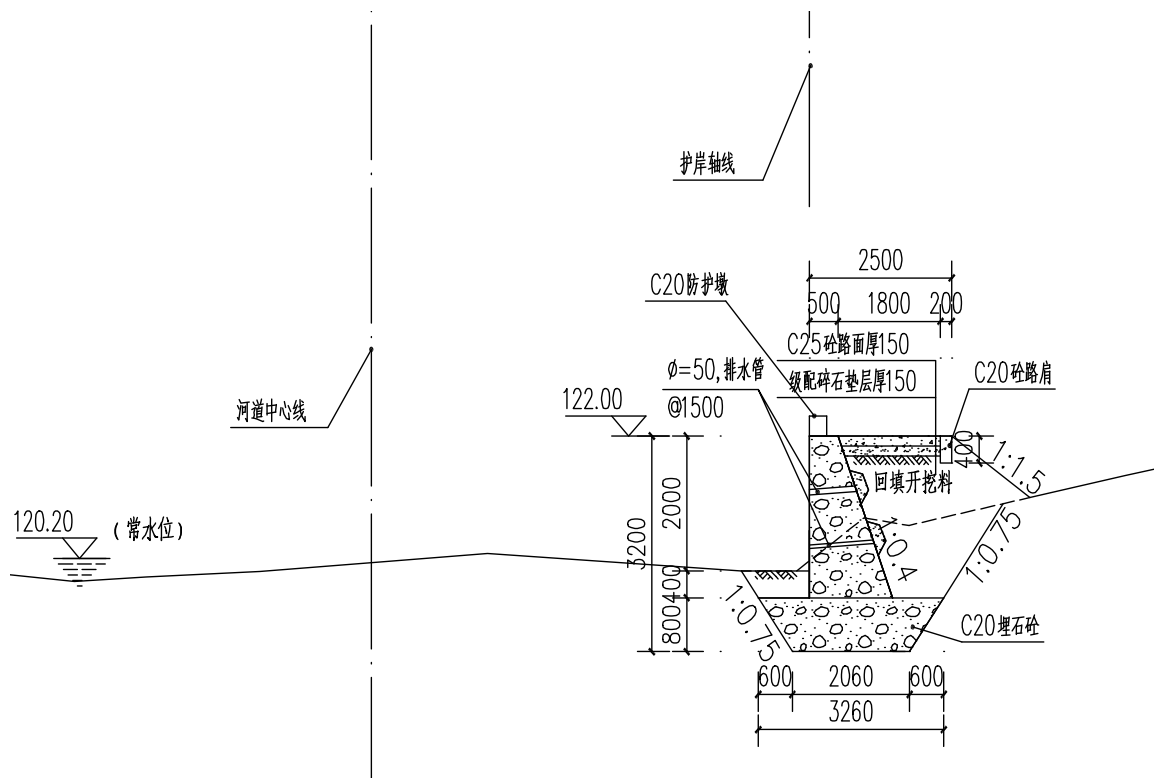
图 2.3-2 代表断面二
