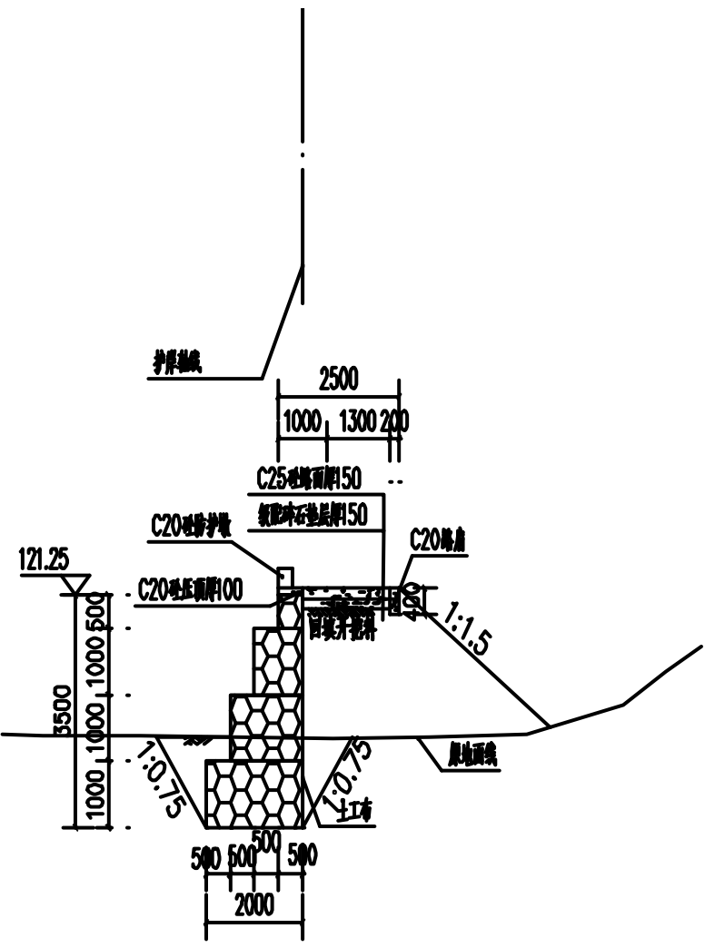
格宾网石笼挡墙典型断面
