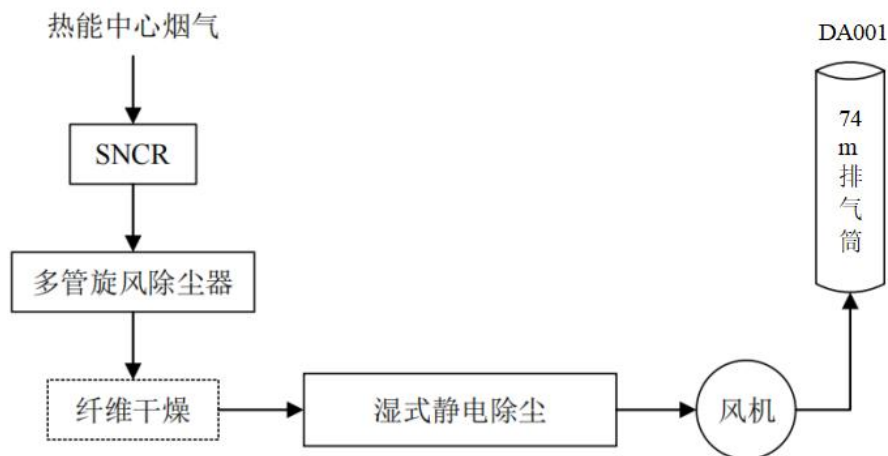
图 5.2-1 热能中心尾气处理工艺流程图
