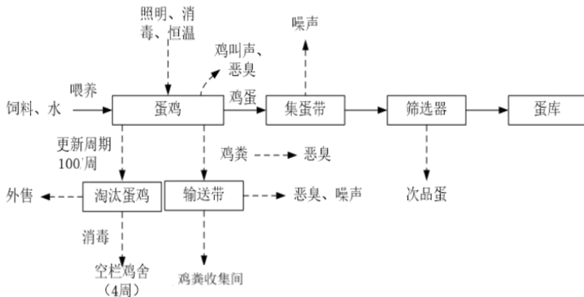
图 2.3.2-1：项目蛋鸡养殖工艺及产排污环节图
