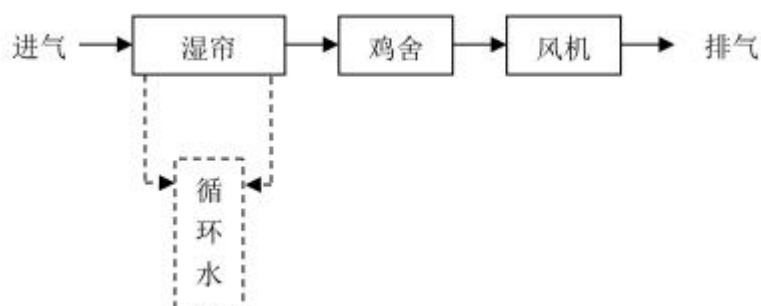
图 2.2-1 水帘通风系统示意图
