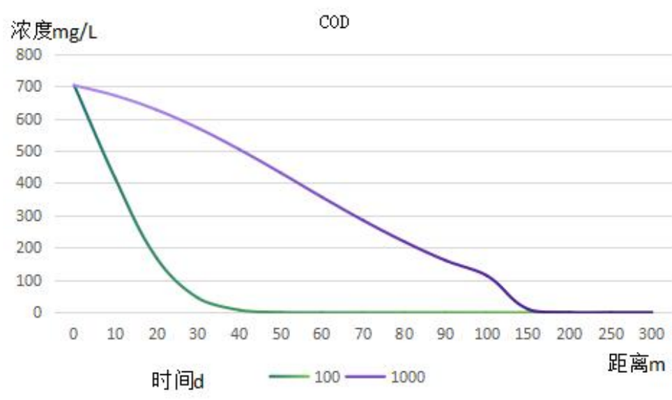
图 4.2.3-2 COD 固定时间（100d、1000d）泄漏后下游地下 0~300m 处浓度分布
