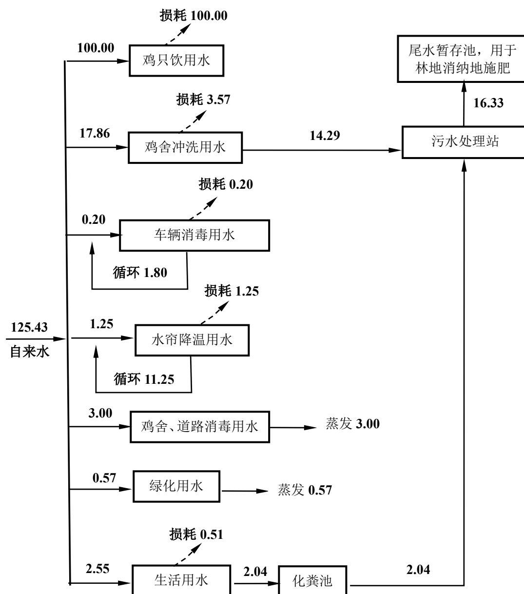
图 2.2-2: 项目水平衡图 单位: m 3 /d
