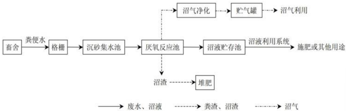
图 5.2.2-1 模式 I 工艺基本流程图
