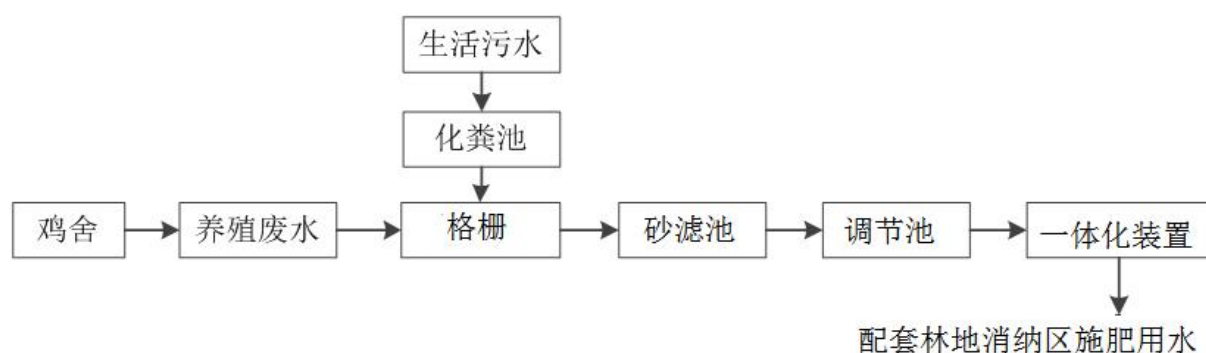
图 2.3.2-2：项目污水处理工艺流程图
