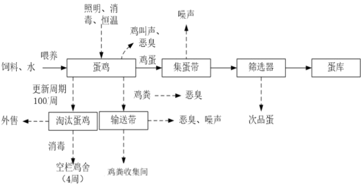
图 2.1-1：现有项目蛋鸡养殖工艺及产排污环节图
