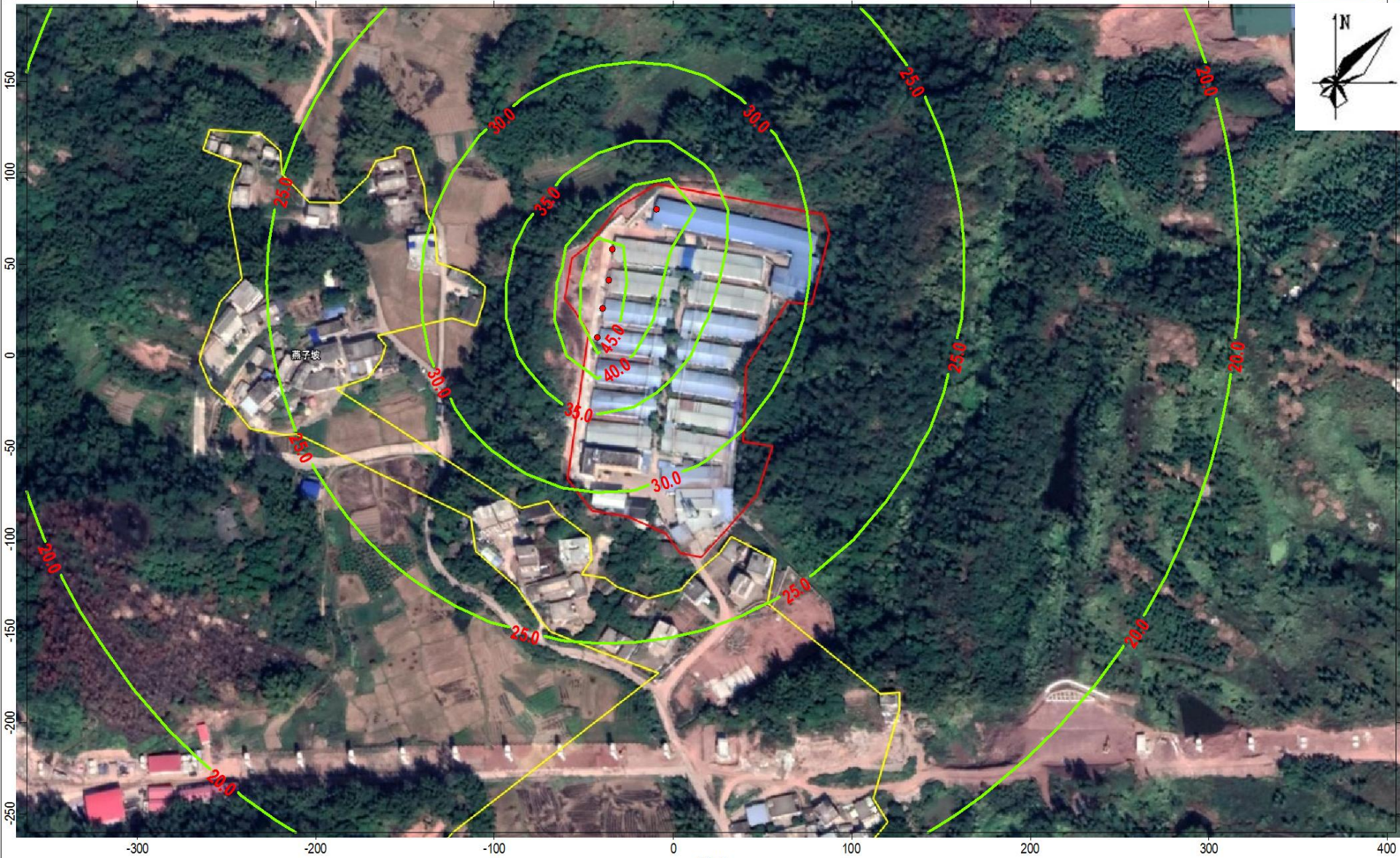
图 4.2.4-2 营运期项目排放噪声贡献值等声级线图（夜间） 单位：dB(A)
