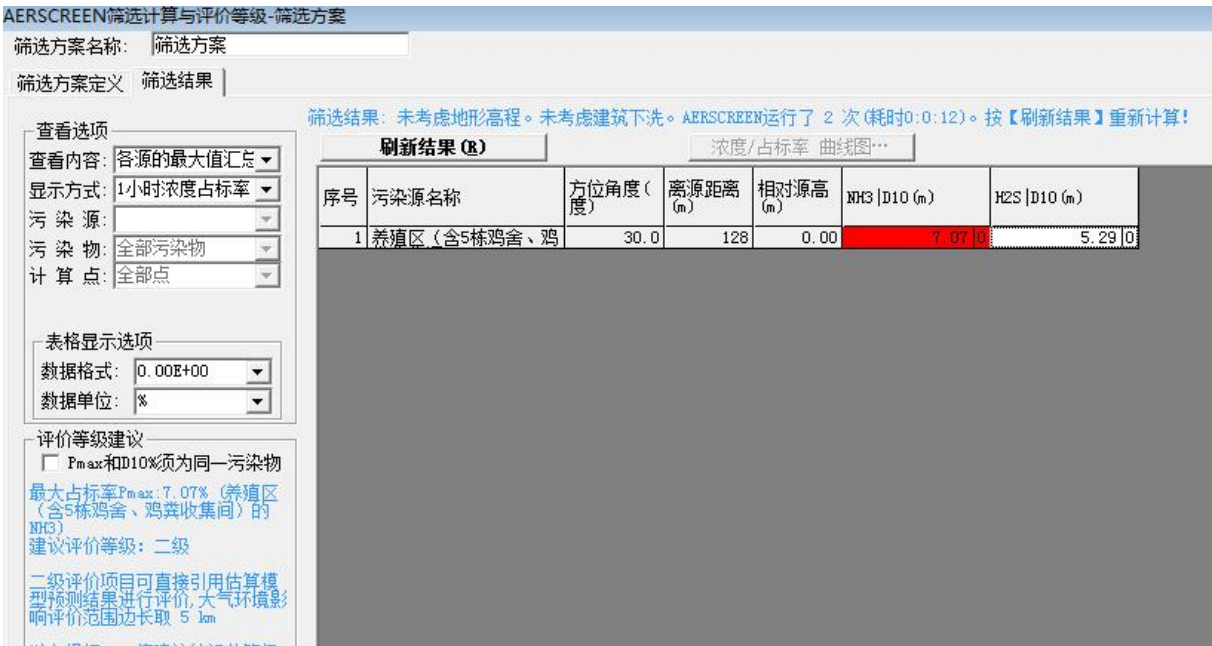
图 4.2.1-1 AERSCREEN 预测结果图
