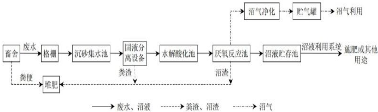
图 5.2.2-2 模式 II 工艺基本流程图
