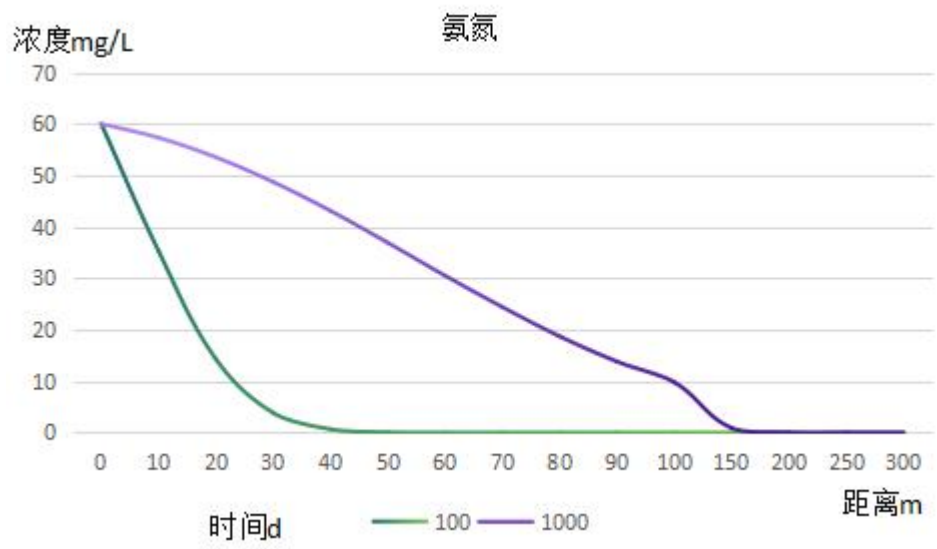
图 4.2.3-3 氨氮固定时间（100d、1000d）泄露后下游地下 0~300m 处浓度分布
