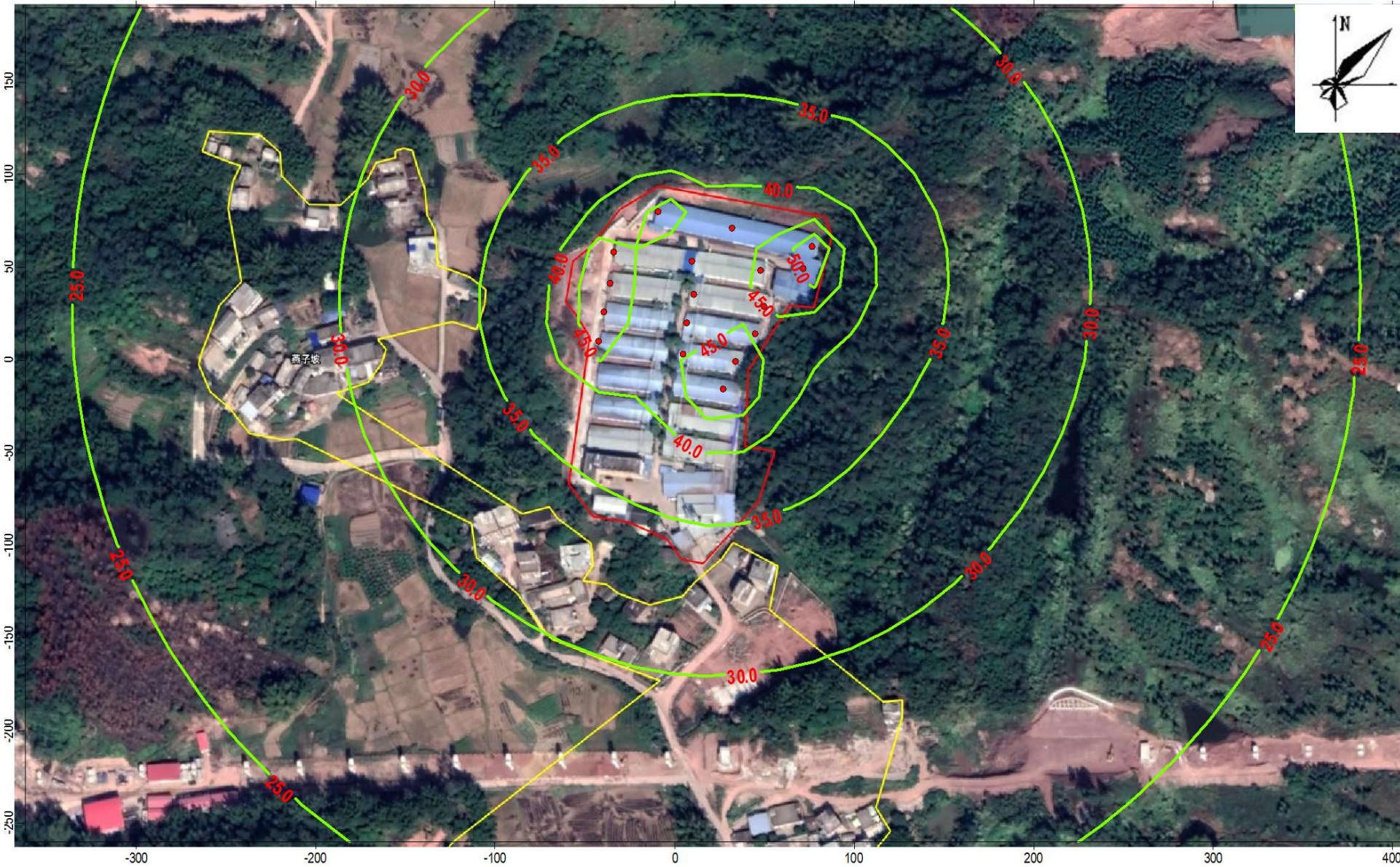
图 4.2.4-1 营运期项目排放噪声贡献值等声级线图（昼间） 单位：dB(A)
