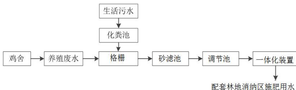
图 5.2.2-4：项目污水处理工艺流程图
