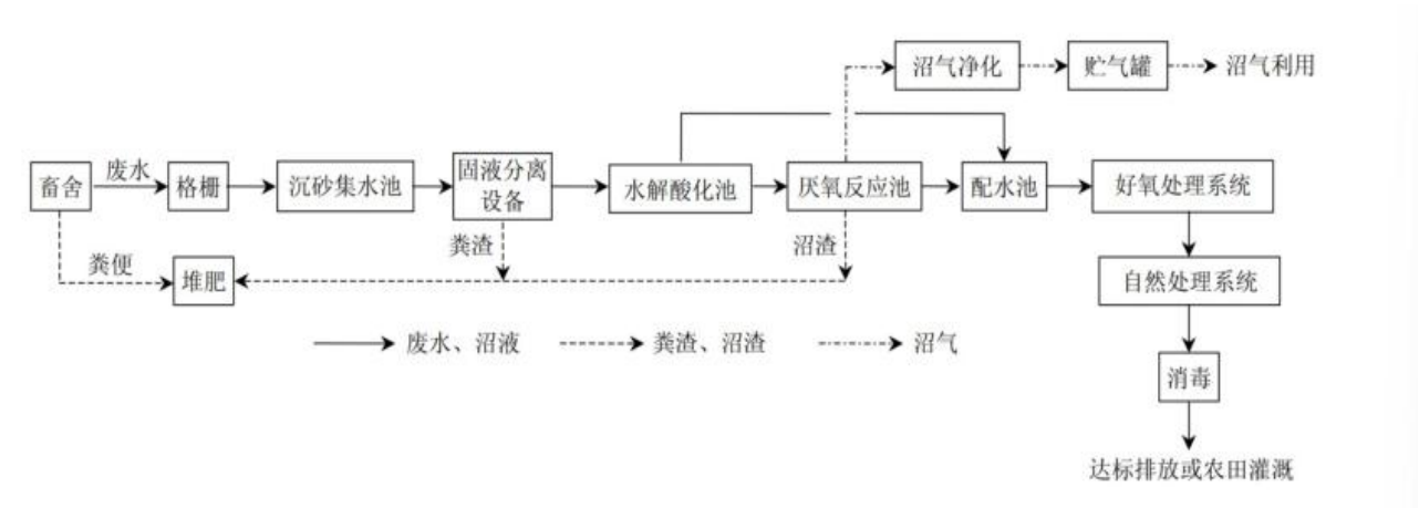
图 5.2.2-3 模式 III 工艺基本流程图
